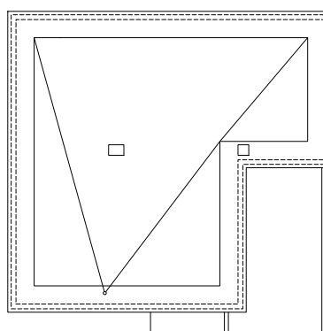
TLOCRT KROVA
