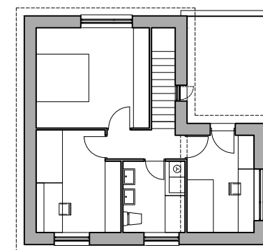
TLOCRT KATA
