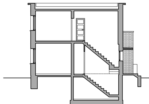
PRESJEK
