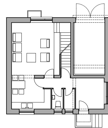
TLOCRT PRIZEMLJA
