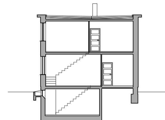
PRESJEK
