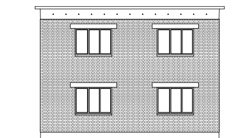
SJEVEROISTOČNO PROČELJE
