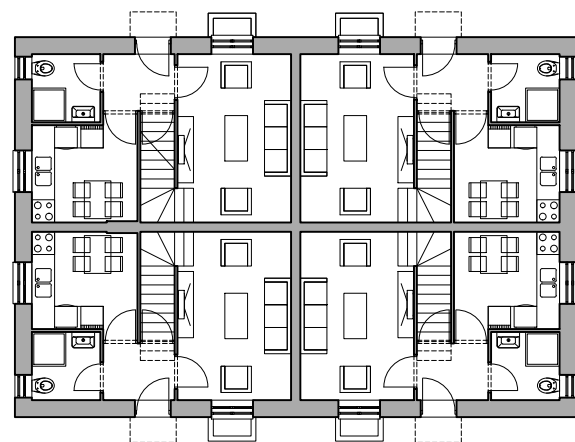
TLOCRT PRIZEMLJA
