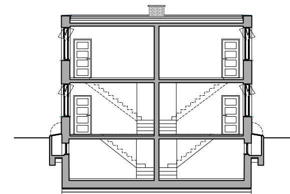
POPREČNI PRESJEK
