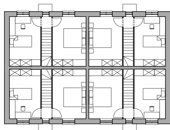
TLOCRT KATA
