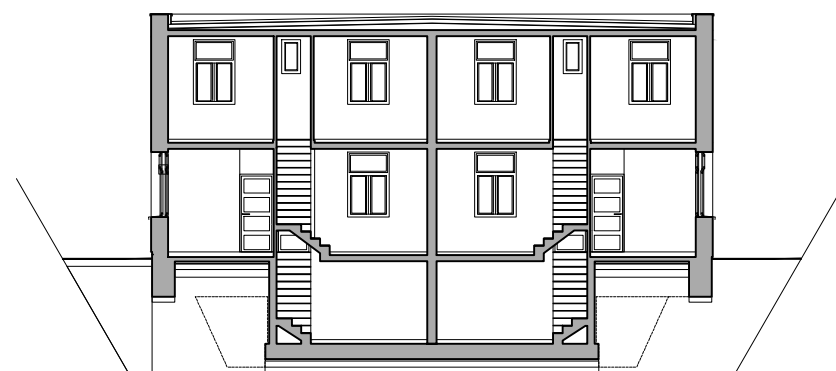
UZDUŽNI PRESJEK
