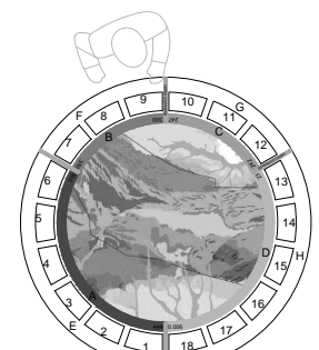
DETALJ_VRSTE STIJENA
