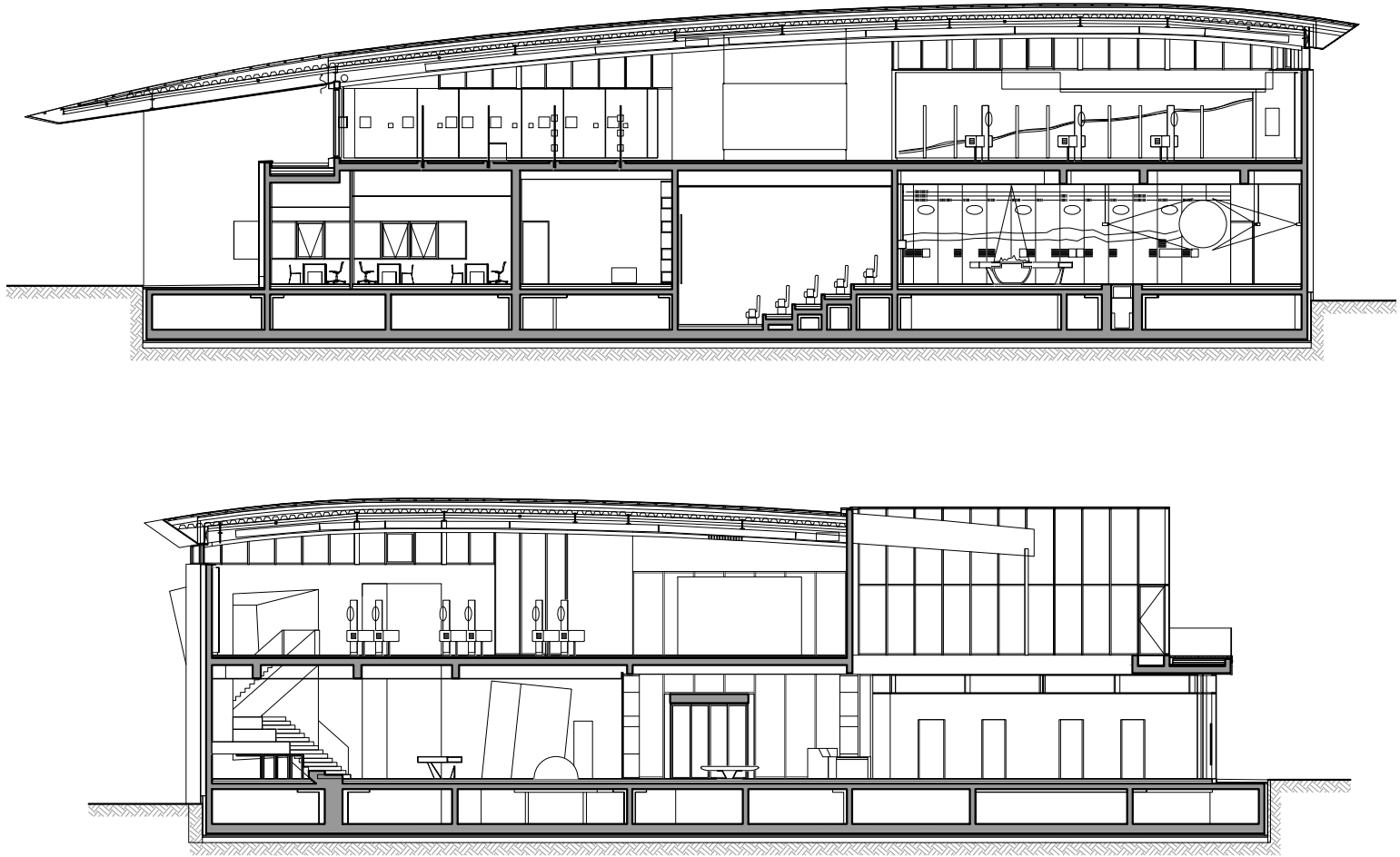
PRESJECI
