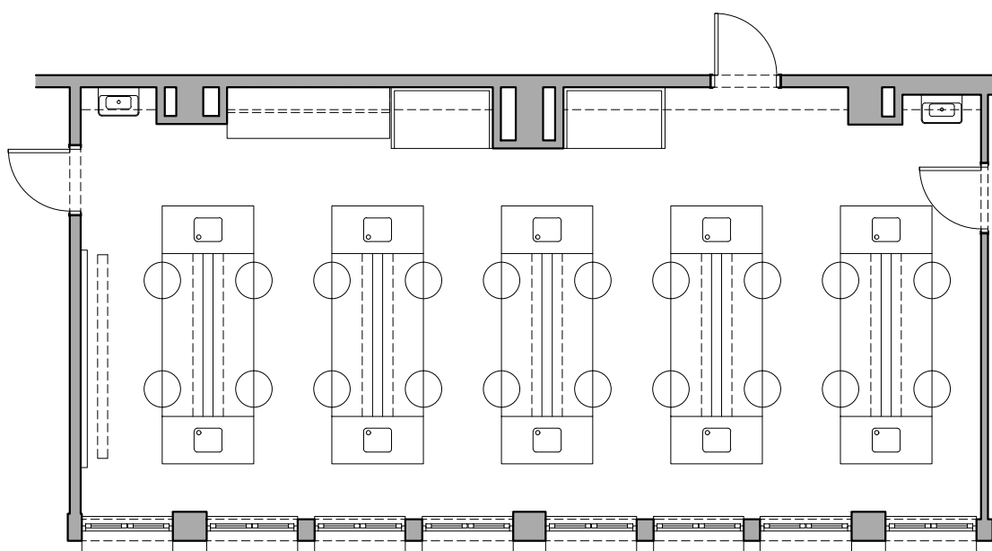
PAVILJON 3_STUDENSKI PRAKTIKUM IZ KEMIJE_TLOCRT
