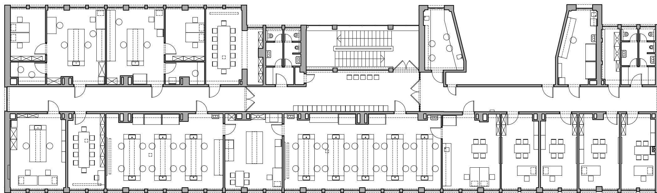
PAVILJON 3_TLOCRT 2. KATA
