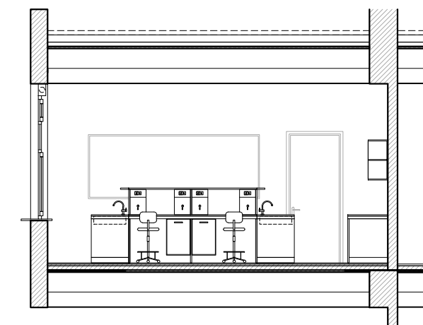
PAVILJON 3_STUDENSKI PRAKTIKUM IZ KEMIJE_POPREČNI PRESJEK
