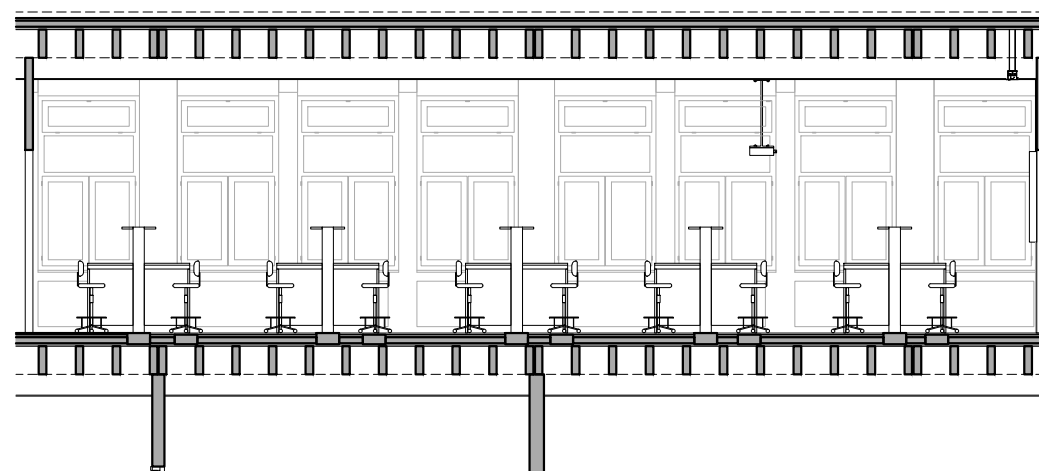
PAVILJON 3_STUDENSKI PRAKTIKUM IZ KEMIJE_UZDUŽNI PRESJEK
